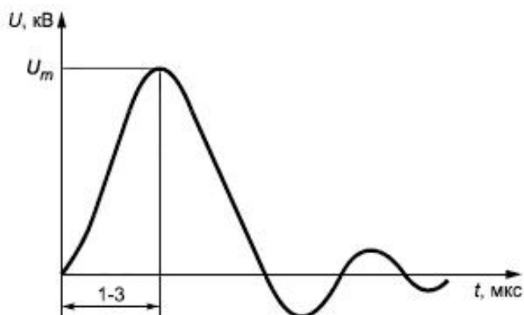
Рисунок Б.2 - Форма импульсов, характерная для точек присоединения a, c, d, e
