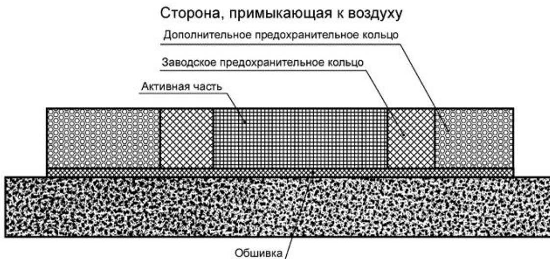
Рисунок 1 - Разрез стационарного тепломера, установленного на испытываемую конструкцию (масштаб по вертикали увеличен)
