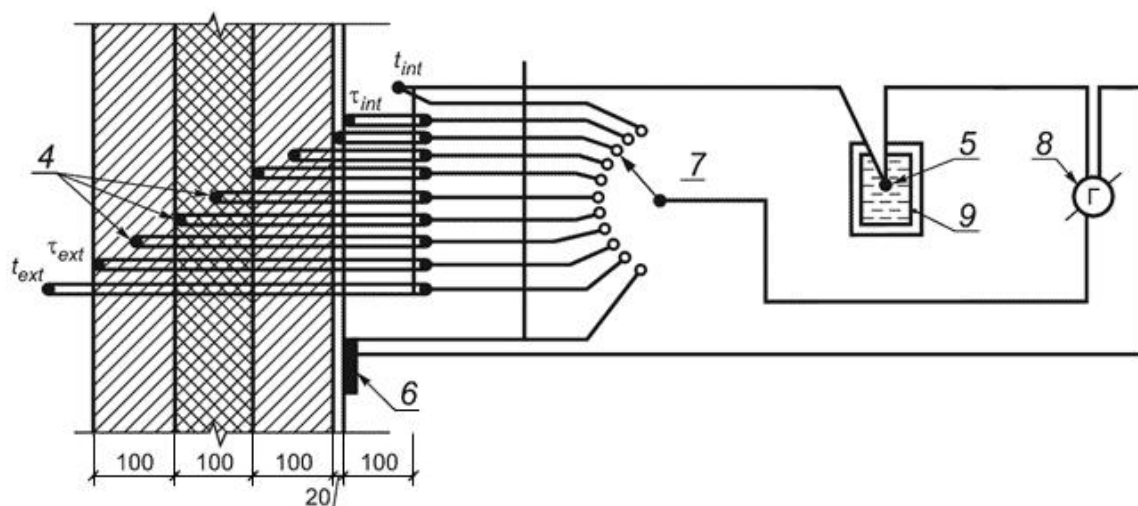
в) Сечение стены и подключение датчиков
