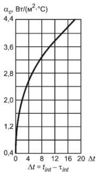
Рисунок Е.1 - График для определения \alpha_c
