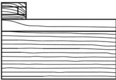
Рисунок 4 - Изотермы ( \delta\theta = 0,05^\circ\text{C} ) для установленного на стене тепломера, обшитого и защищенного (цилиндрическое сечение)
