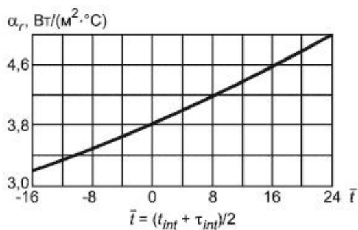
Рисунок Е.2 - График для определения \alpha_\gamma
