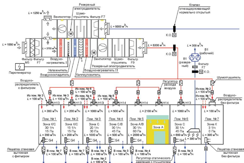
Рисунок Б.1 - Пример принципиальной схемы вентиляции и кондиционирования воздуха
