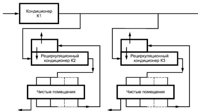
Рисунок А.4 - Двухуровневая система вентиляции и кондиционирования
