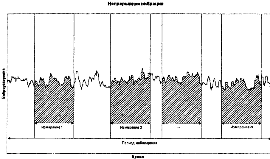
Рис. 2. Периоды контроля, наблюдения и измерений в случае непрерывной вибрации
